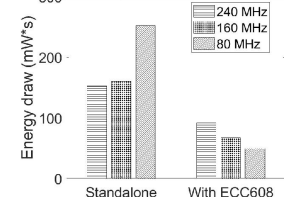
Fig. 14: ECDSA sig. gen. energy draw.
